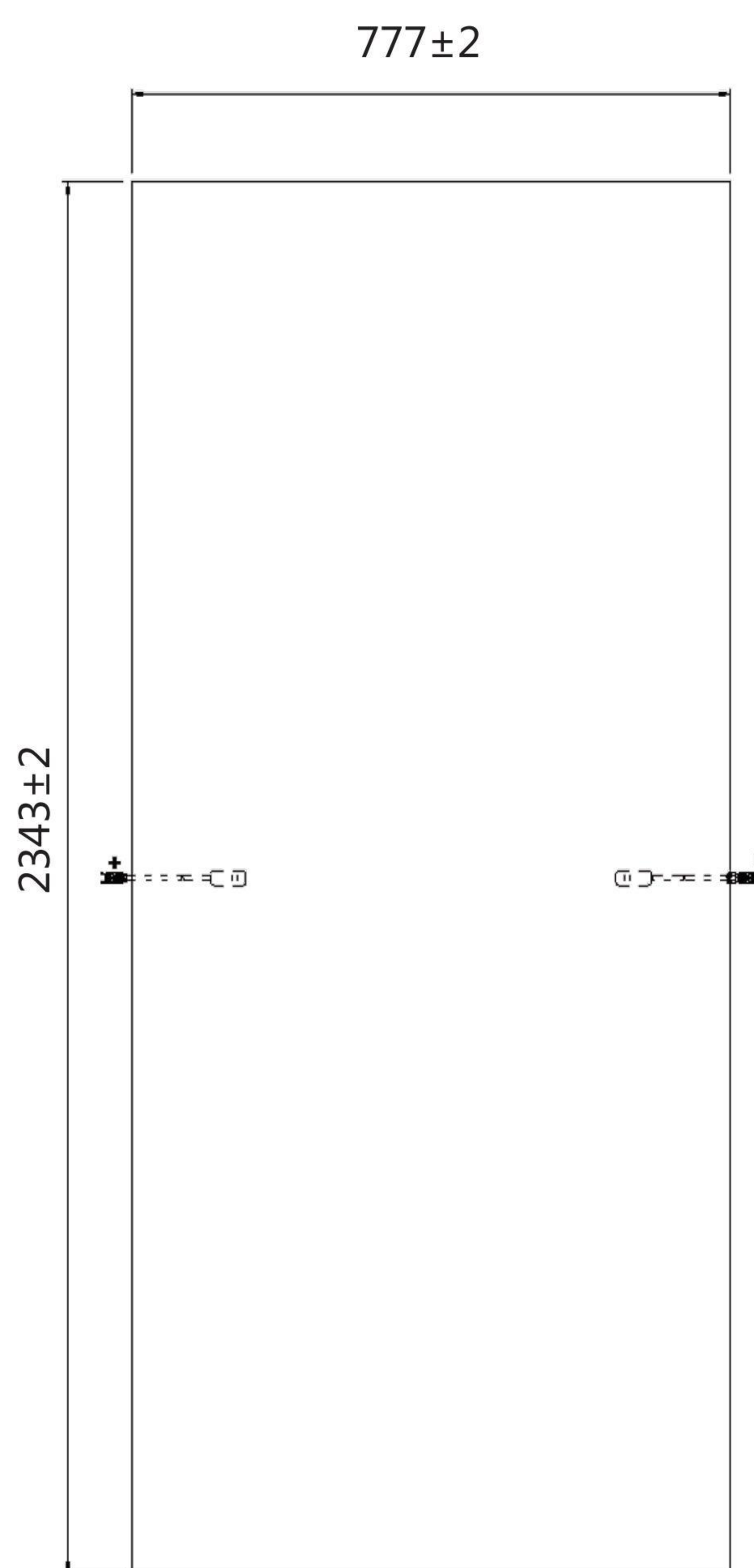
PV module dimensions (mm)
