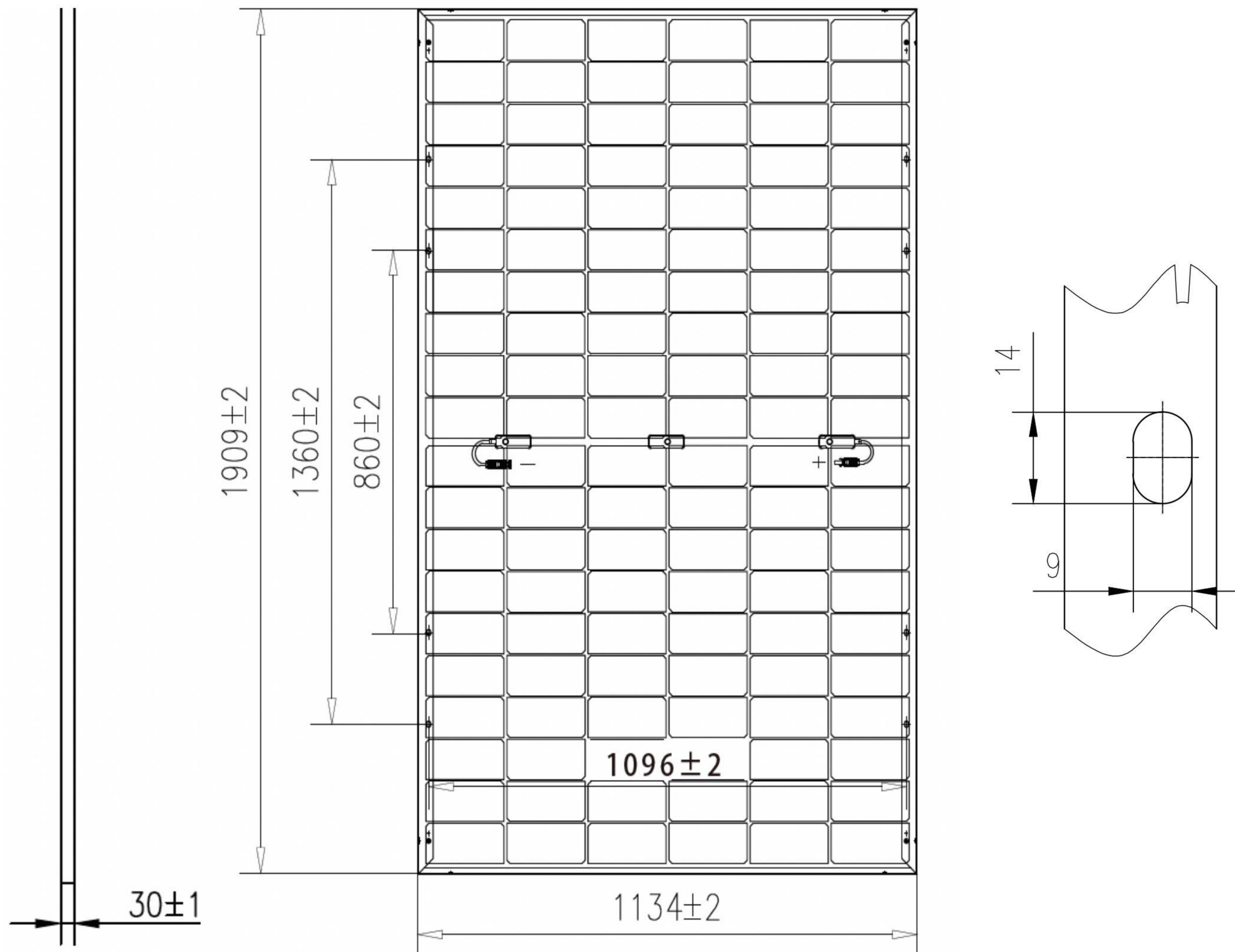
PV module dimensions (mm)
